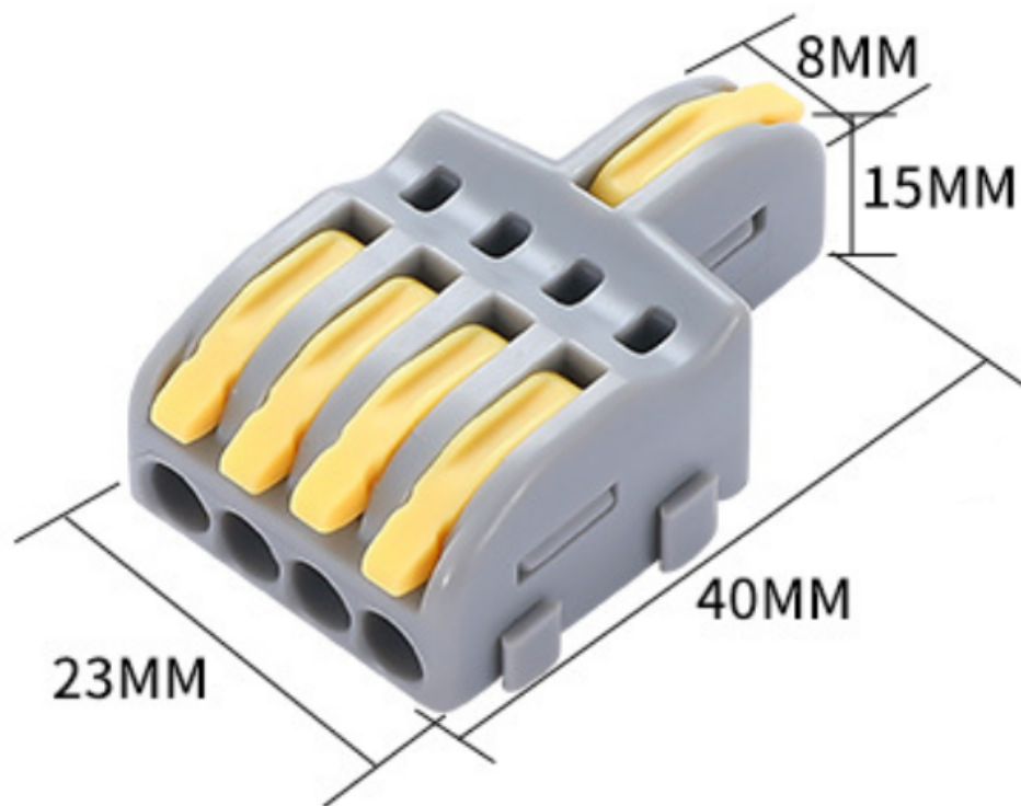
一进四出黄色接线端子
